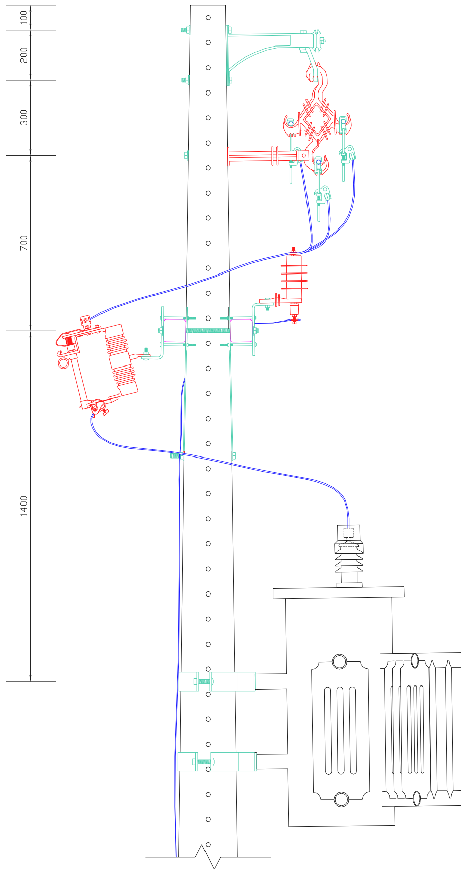
Instalação padrão para transformadores
