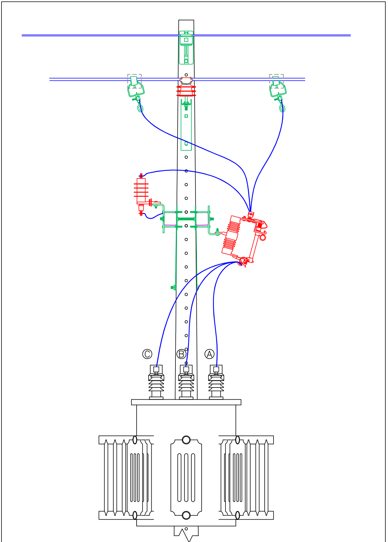
Instalação padrão para transformadores
