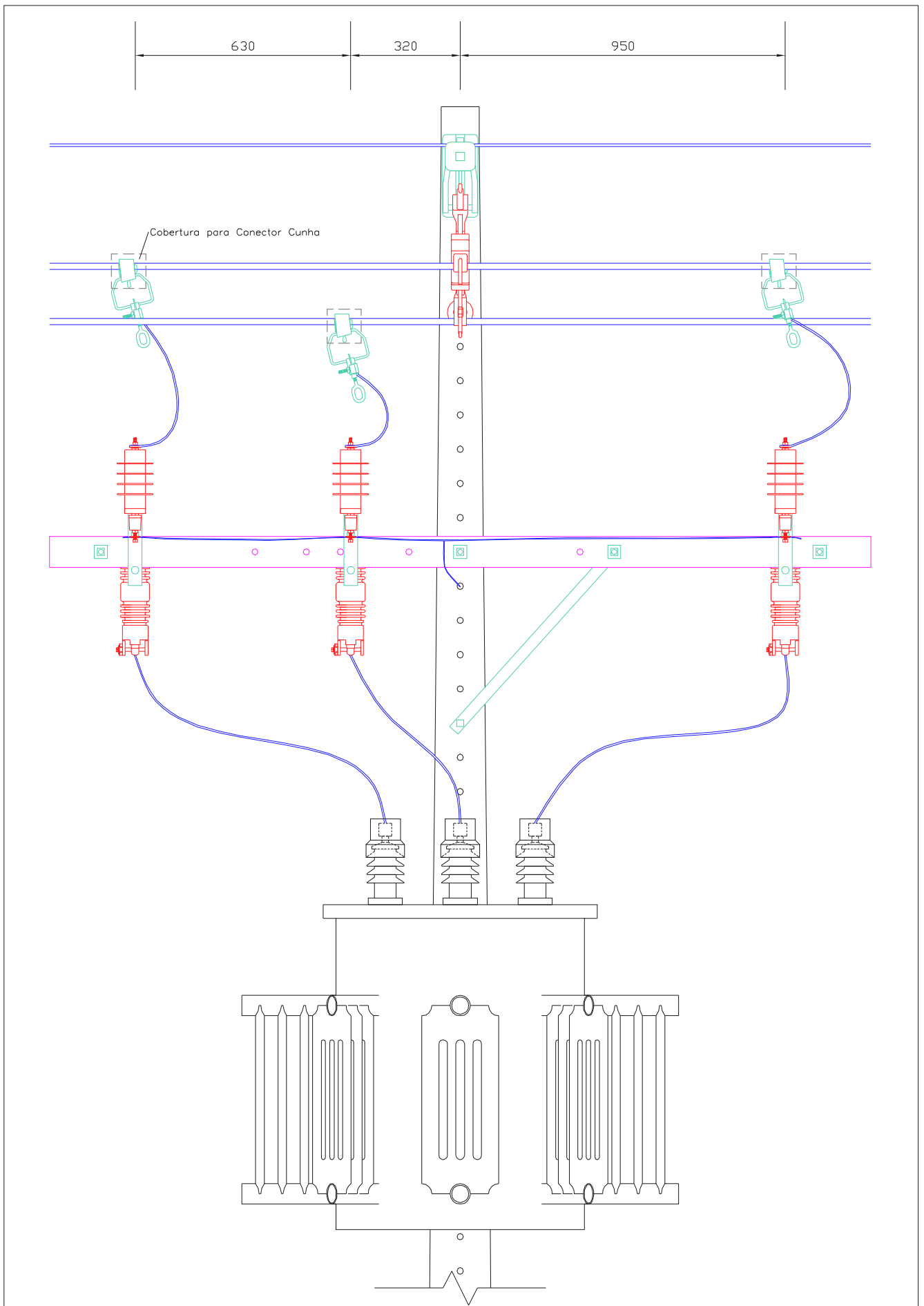
Instalação padrão para transformadores
