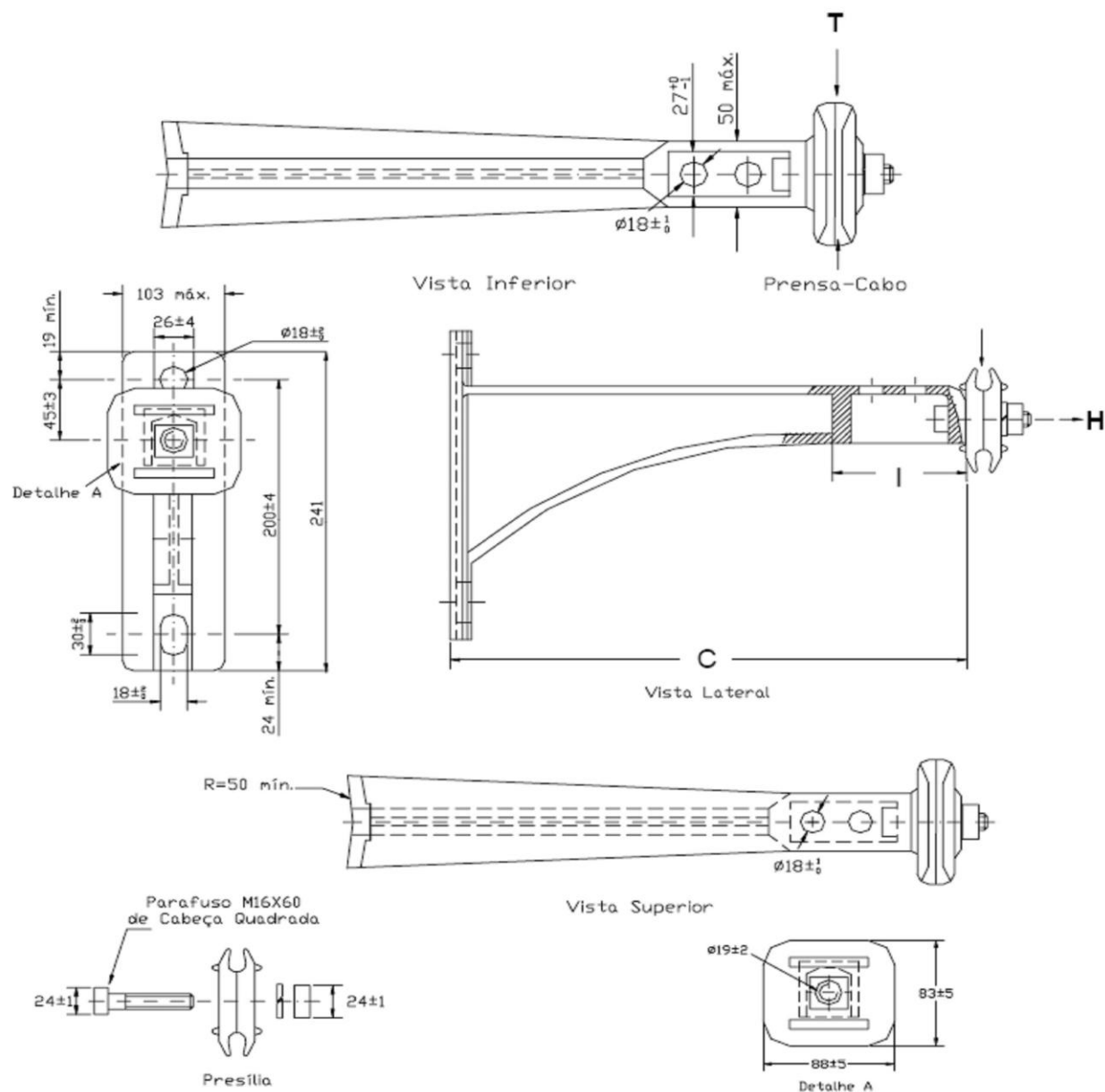
Desenho Item 1.16 do Termo de Referência – código 197 – Braço Tipo L
